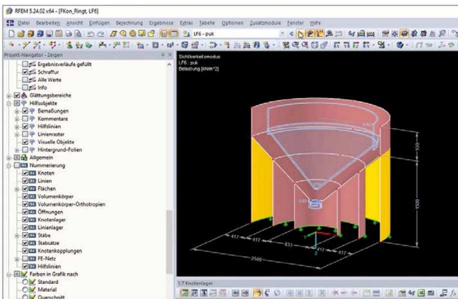
Beispiel: Export der Berechnungsdaten für einen konischem Boden in eine FEM-Umgebung:
