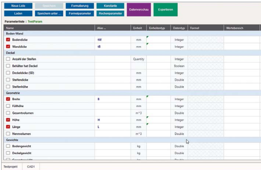
Parameterauswahlfenster
